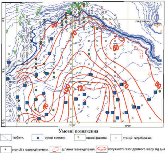
Рис. 3. Розрахунок BSR – межі стійкості газогідратів у глибині осадів
